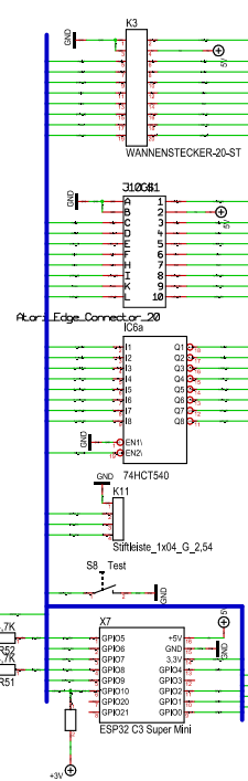
J10 Aux
